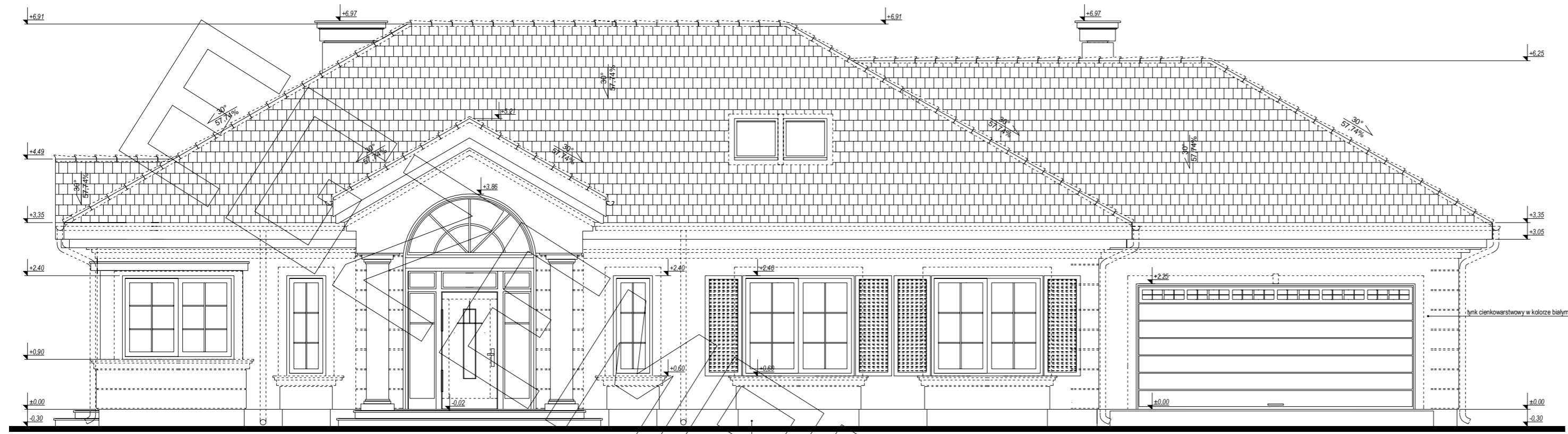
ELEWACJA FRONTOWA:
